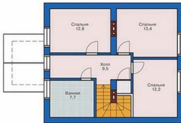
План мансардного этажа
